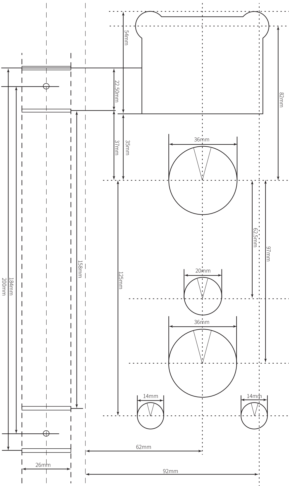
芝麻云锁 (6298锁体) 开孔图
